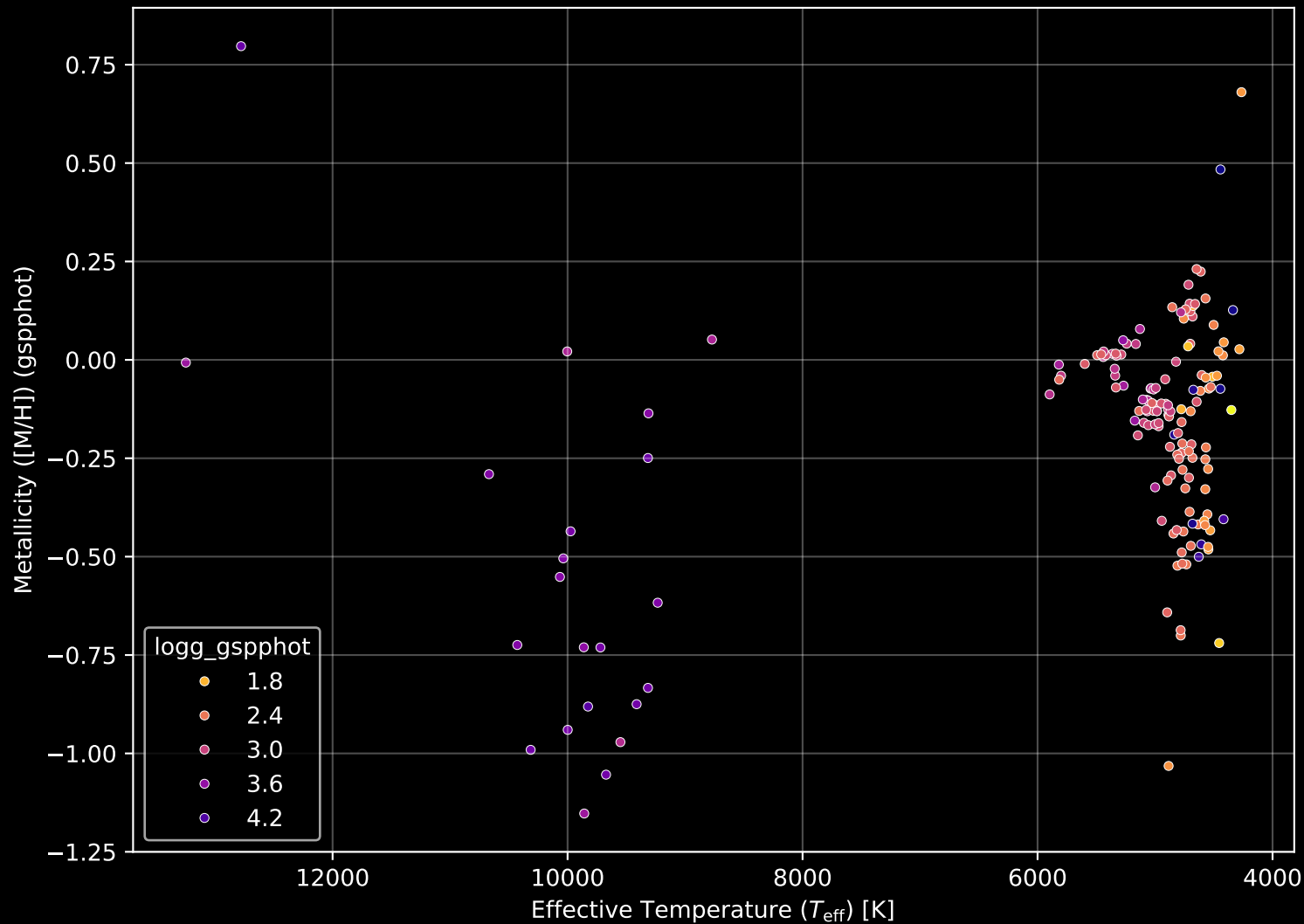
APOGEE DR17 Field: [235+06] Stellar Population Parameters (n= 159)
